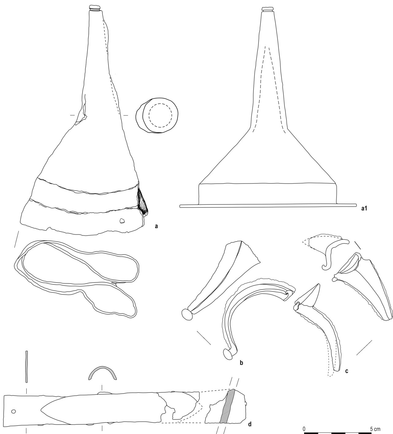
Ryc. 1. Rzeszów - Zalesie. Część inwentarza grobu. a-d – żelazo (a1 – rekonstrukcja umba). Rys.: A. Kokowski i A. Jączek Fig. 1. Rzeszów - Zalesie. Part of a grave equipment. a-d – iron (a1 – reconstruction of the shield boss). Drawing: A. Kokowski & A. Jączek
