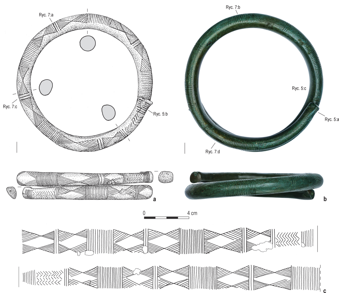
Ryc. 4. Siwianka, pow. otwocki. Nagołennik 1. Rys.: B. Karch (a, c). Fot.: B. Solarewicz (b)
