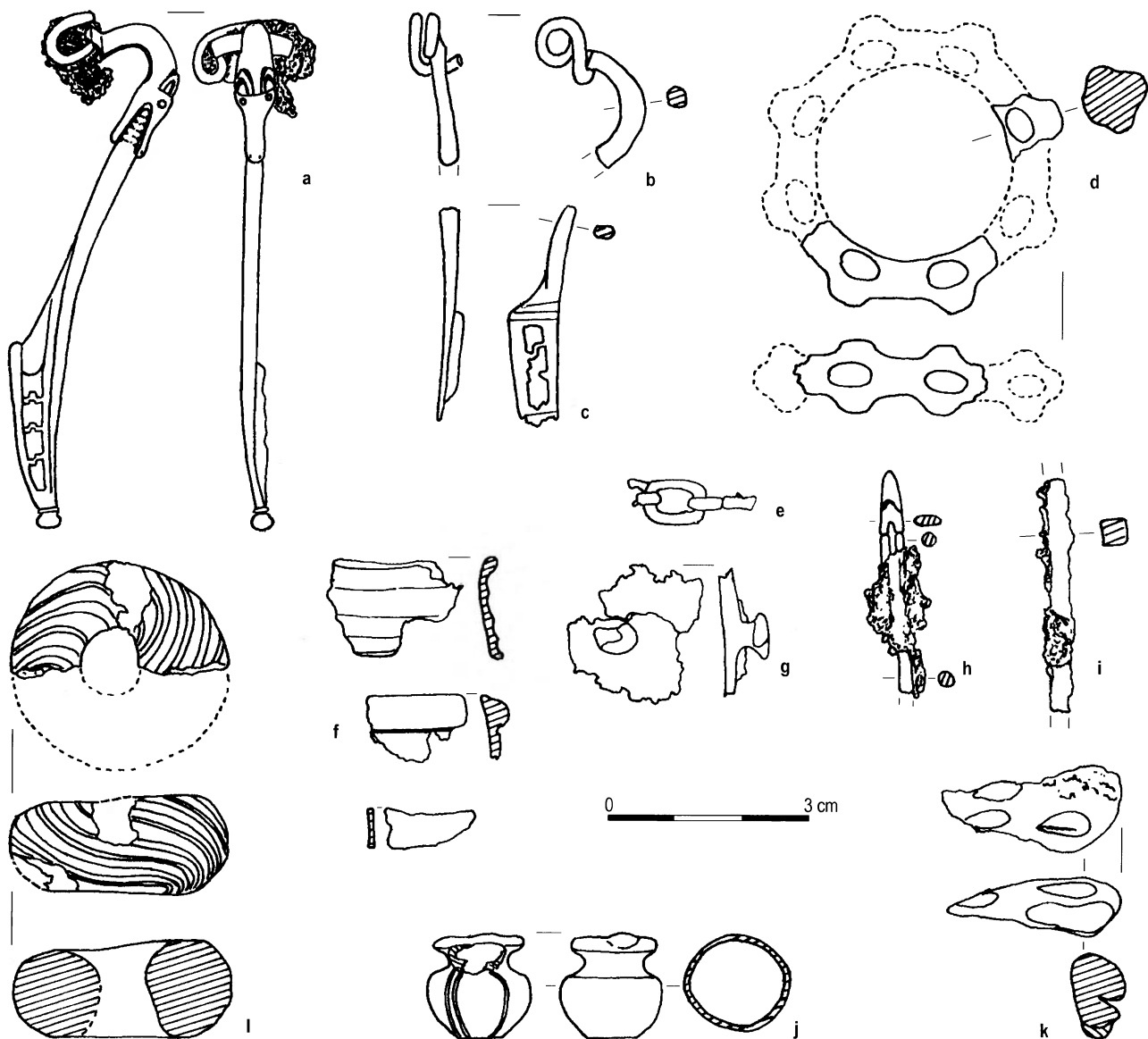
Ryc. 2. Podwiesiek stan. 2(?), woj. kujawsko-pomorskie. Wybór zabytków. Brąz (a–f), żelazo (g–i), szkło (j–l)
