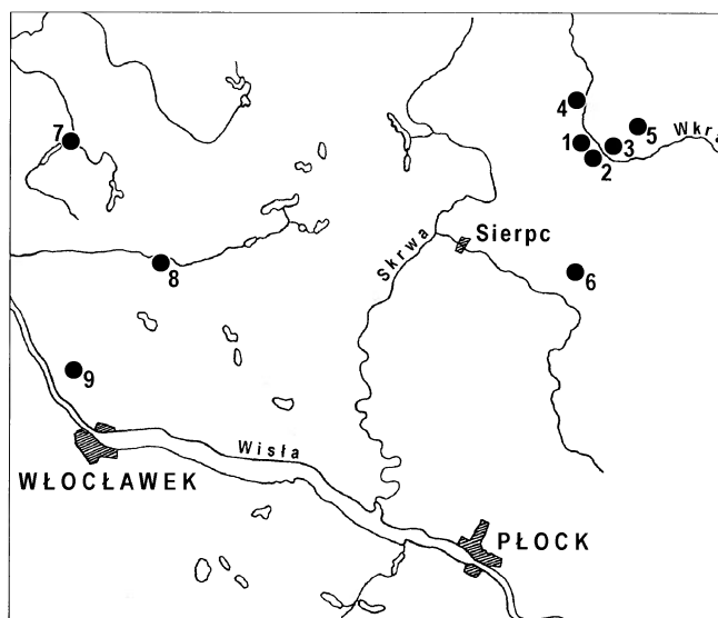
Ryc. 1. Stanowiska późnopaleolityczne i mezolityczne z badań F. Tarczyńskiego (numery na mapie odpowiadają numerom stanowisk w tekście)
