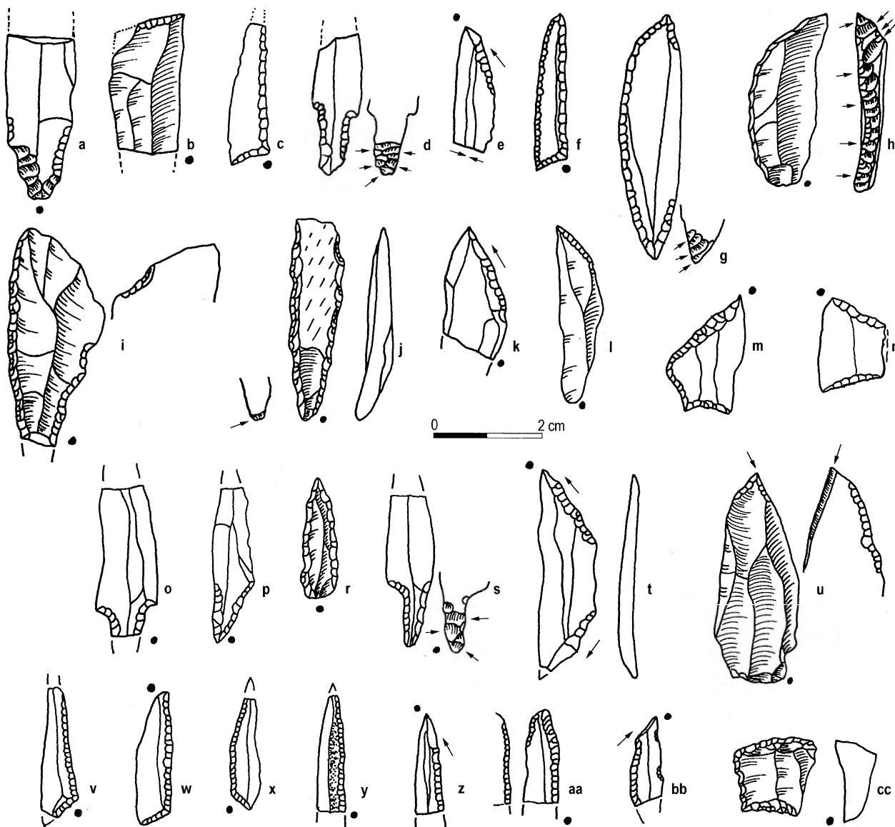
Ryc. 3. Sławęcino (a); Przytulewo (b); Zawidz Kościelny (i–cc), woj. mazowieckie; Hornówek (c); Lipno (d–f); Winduga–Rachcin (g), woj. kujawsko-pomorskie
