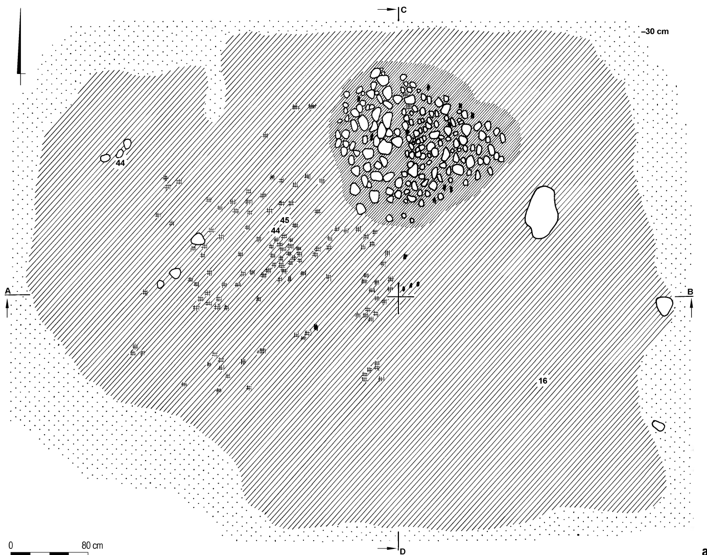
Ryc. 7.1. Łęgonice, pow. Grójec, stan. 1. Chata 3: plany (a, c) i profile obiektu (b) oraz dołków posłupowych (d) Fig. 7.1. Łęgonice, distr. Grójec, site 1. Hut 3: plans (a, c) and cross-sections of the hut (b) and post-holes (d)
