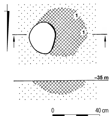
Ryc. 27. Łęgonice, pow. Grójec, stan. 1. Plan i profil jamy 60
