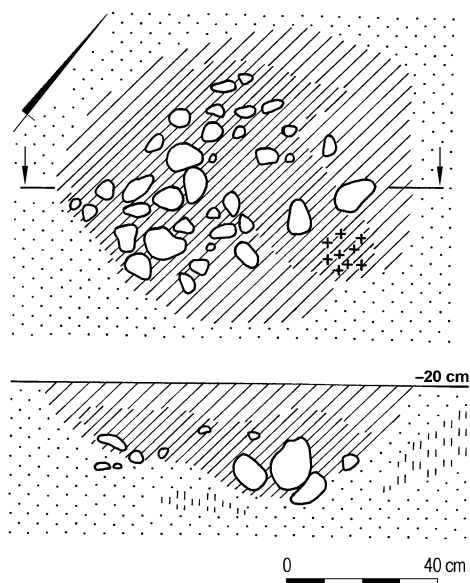
Ryc. 30. Łęgonica, pow. Grójec, stan. 1. Plan i profil jamy 80
