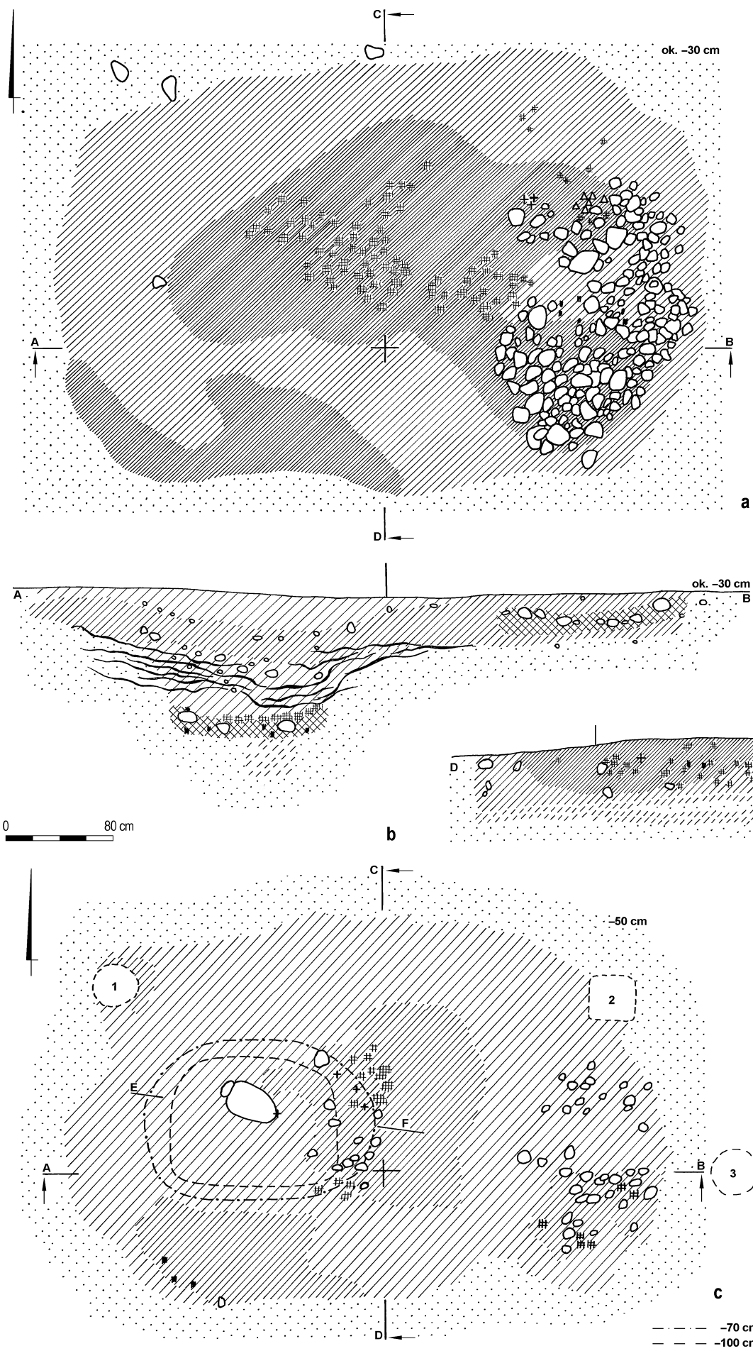
Ryc. 9.1. Lęgonice, pow. Grójec, stan. 1. Chata 4: plany wraz z zarysami dołków posłupowych i jamy (a, c) i profile obiektu (b) oraz plany i profil jamy (d) Fig. 9.1. Lęgonice, distr. Grójec, site 1. Hut 4: plans with outlines of post-holes and pit (a, c), cross-sections of the hut (b) and plan and cross-section of pit (d)
