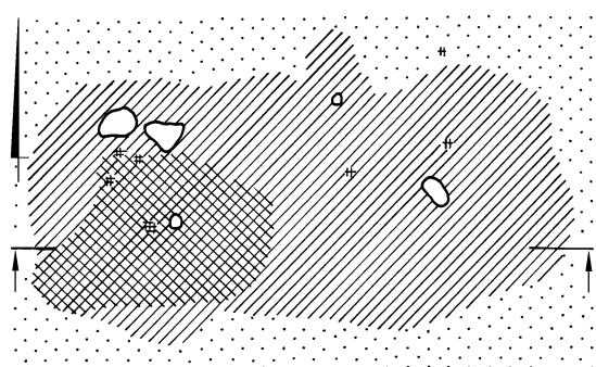
Ryc. 35. Łęgonicze, pow. Grójec, stan. I. Plan i profil skupiska polepy 2 Fig. 35. Łęgonicze, distr. Grójec, site I. Plan and cross-section of daub concentration 2
