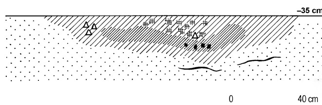
Ryc. 35. Łęgonicze, pow. Grójec, stan. I. Plan i profil skupiska polepy 2 Fig. 35. Łęgonicze, distr. Grójec, site I. Plan and cross-section of daub concentration 2
