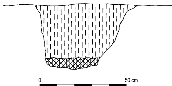
Ryc. 9. Transbór, pow. Mińsk Maz. Profil obiektu 9
