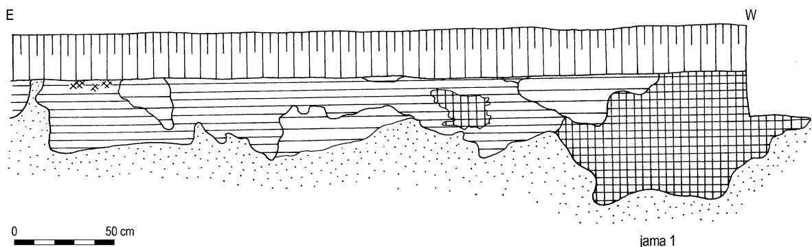
Ryc. 16. Transbór, pow. Mińsk Maz. Profil W-E obiektu 15 (jamy 1) Fig. 16. Transbór, Mińsk Maz. Cross-section W-E of feature 15 ('pit 1')
