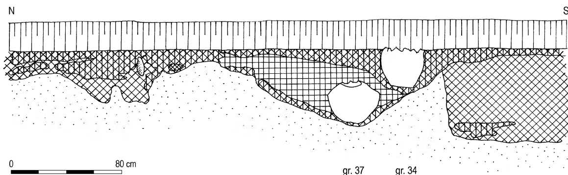
Ryc. 25. Transbór, pow. Mińsk Maz. Profil N-S obiektu 21 Fig. 25. Transbór, distr. Mińsk Maz. Cross-section N-S of feature 21
