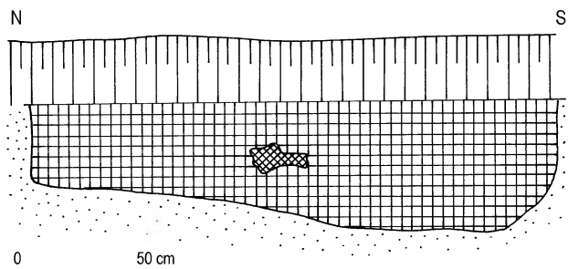
Ryc. 17. Transbór, pow. Mińsk Maz. Profil N-S obiektu 15 (jamy 1) Fig. 17. Transbór, distr. Mińsk Maz. Cross-section N-S of feature 15 ('pit 1')
