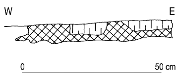
Ryc. 38. Transbór, pow. Mińsk Maz. Profil pasów podłużnych. Odcinek IV/9
