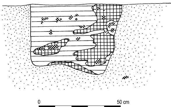
Ryc. 11. Transbór, pow. Mińsk Maz. Profil obiektu 12 Fig. 11. Transbór, distr. Mińsk Maz. Cross-section of feature 12
