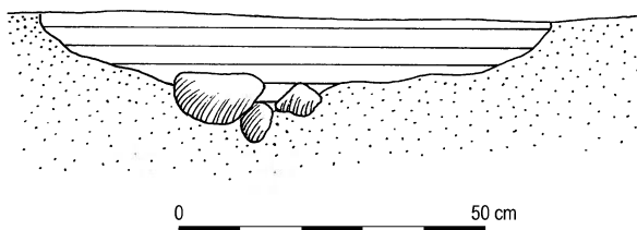
Ryc. 12. Transbór, pow. Mińsk Maz. Profil obiektu 13 Fig. 12. Transbór, distr. Mińsk Maz. Cross-section of feature 13
