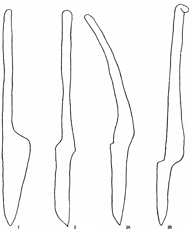
Ryc. 2. Różne typy noży wykuwanych w okresie wikingim w Danii (por. ryc. 1). 1 – nóż z prostym grzbietem i "wiszącym" ostrzem, 2 – różne noże z trzpieniem wyprowadzonym pośrodku ostrza. Rys. A. Lundgren
