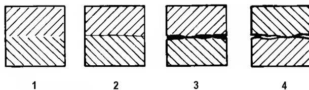
Ryc. 3. Schemat zgrzewów noży żelaznych z Danii:
