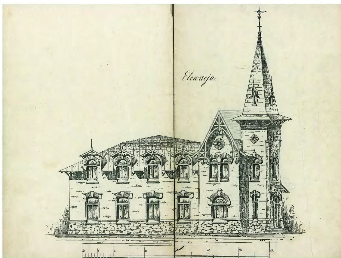
Ryc. 55. Projekt elewacji budynku przy ul. Langnerowskiej w Warszawie wykonany przez Oskara Sosnowskiego w 1912 r. Archiwum PMA Fig. 55. Design of the elevation of a building at Langnerowska St. in Warsaw developed by Oskar Sosnowski in 1912. PMA Archive
