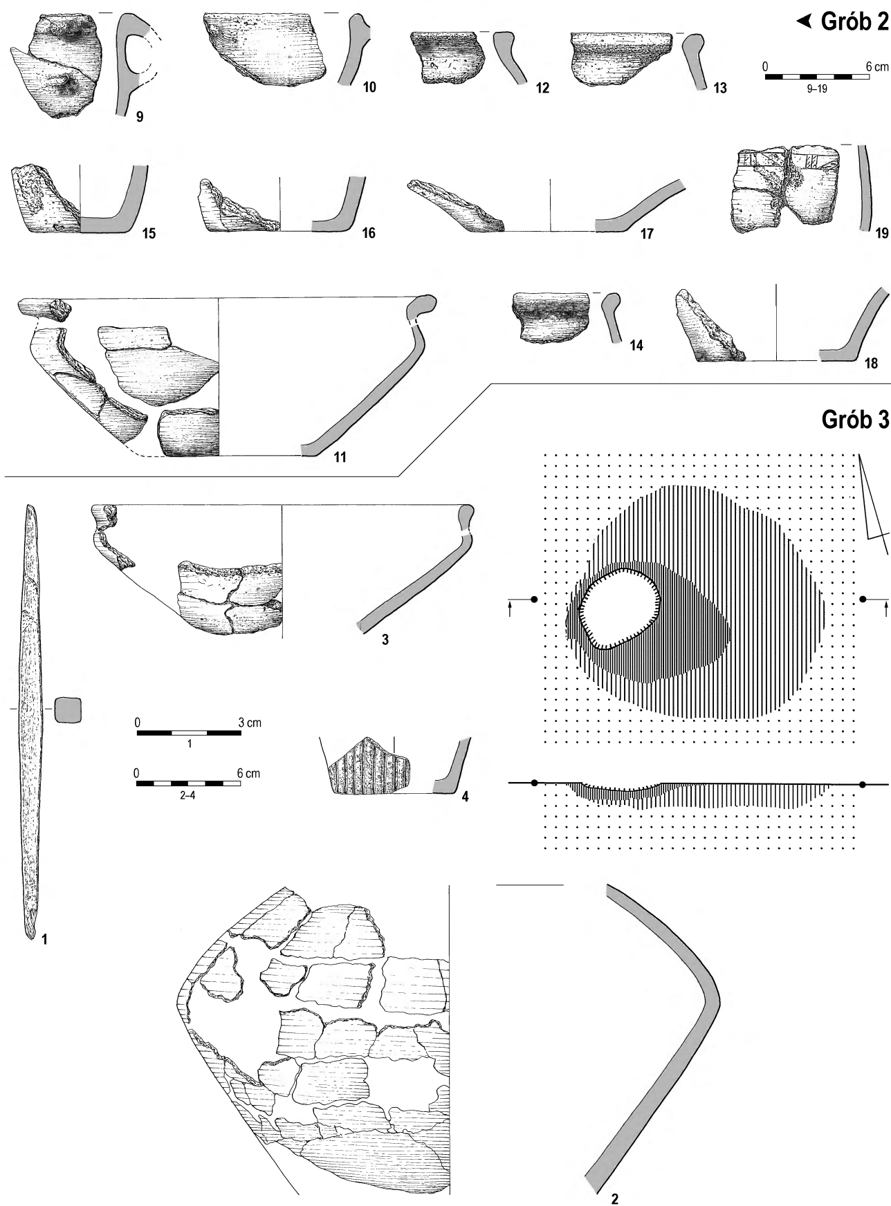
Tabl. III. Całowanie, pow. otwocki, stan. XXVI. Groby 2 i 3. 2:9-19, 3:2-4 – glina; 3:1 – żelazo. Rys. B. Karch Pl. III. Całowanie, distr. Otwock, site XXVI. Graves 2 and 3. 2:9-19, 3:2-4 – pottery; 3:1 – iron. Drawn by B. Karch
