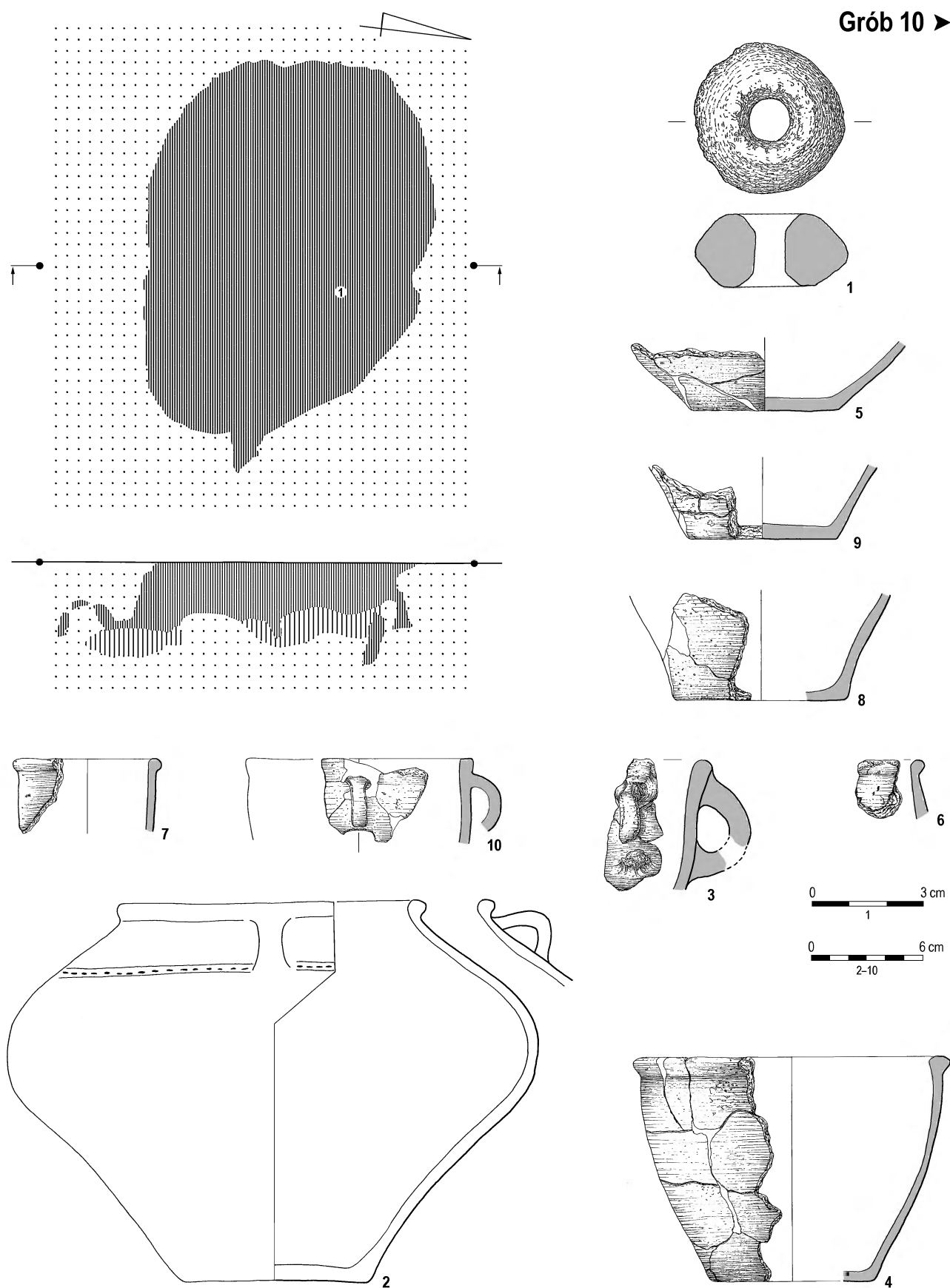
Tabl. VII. Całowanie, pow. otwocki, stan. XXVI. Grób 10. Wszystko glina. Rys. B. Karch Pl. VII. Całowanie, distr. Otwock, site XXVI. Grave 10. Pottery. Drawn by B. Karch
