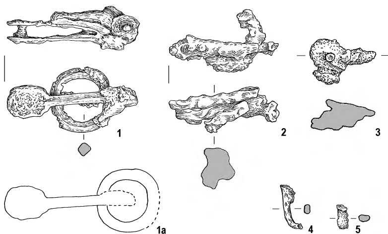
Tabl. VI. Całowanie, pow. otwocki, stan. XXVI. Groby 7, 8 i 9. 7:1.2, 8:1.2, 9:6-9 – glina; 9:1-5 – żelazo. Rys. B. Karch Pl. VI. Całowanie, distr. Otwock, site XXVI. Graves 7, 8 and 9. 7:1.2, 8:1.2, 9:6-9 – pottery; 9:1-5 – iron. Drawn by B. Karch
