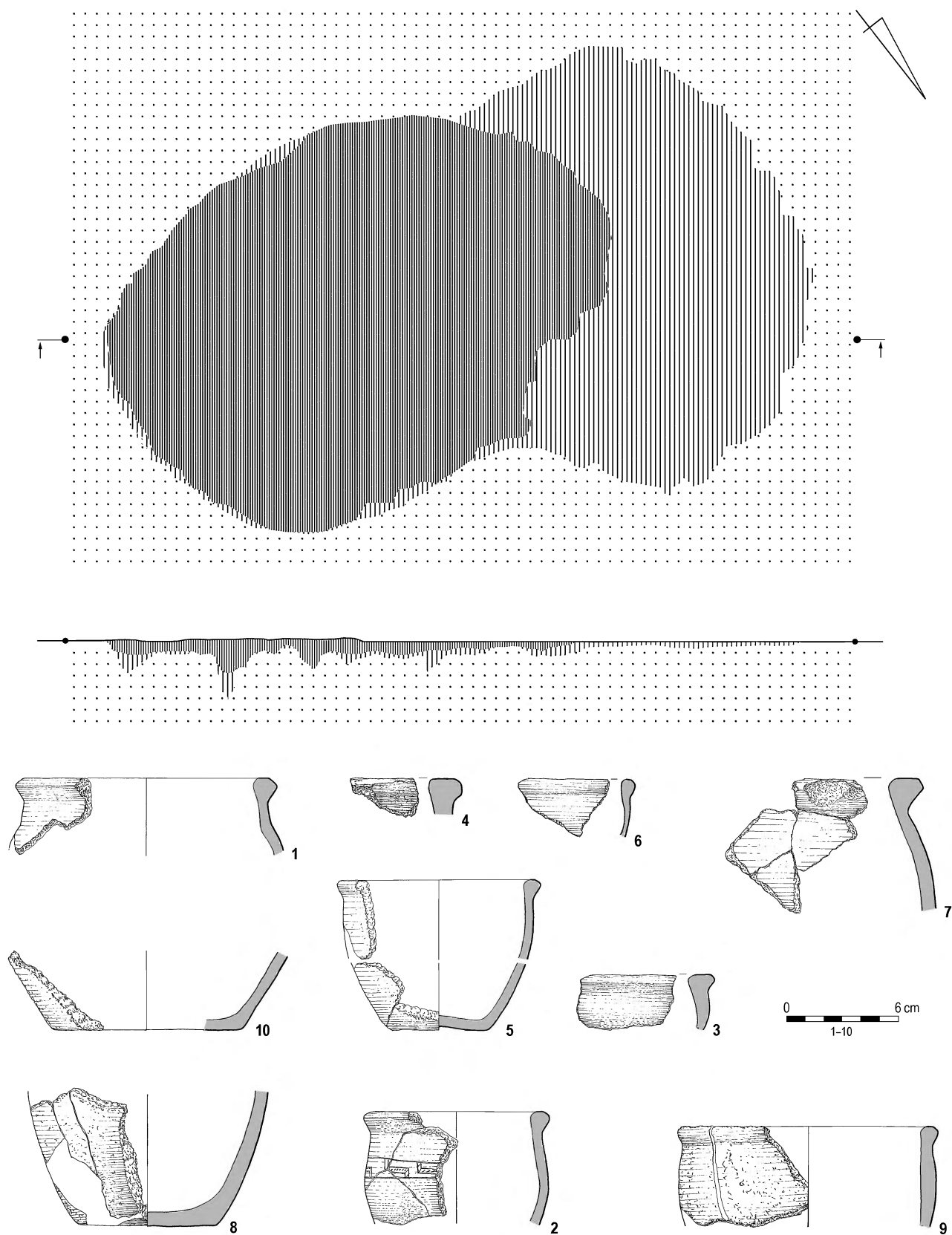
Tabl. X. Całowanie, pow. otwocki, stan. XXVI. Grób 15. Wszystko glina. Rys. B. Karch Pl. X. Całowanie, distr. Otwock, site XXVI. Grave 15. Pottery. Drawn by B. Karch
