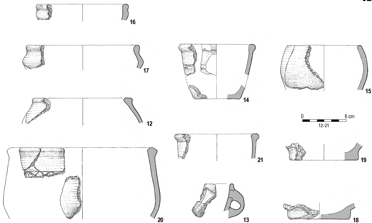
Tabl. XIII. Całowanie, pow. otwocki, stan. XXVI. Zabytki luźne. 01:6-8 – żelazo, pozostałe glina. Rys. B. Karch Pl. XIII. Całowanie, distr. Otwock, site XXVI. Stray finds. 01:6-8 – iron, all other finds – pottery. Drawn by B. Karch
