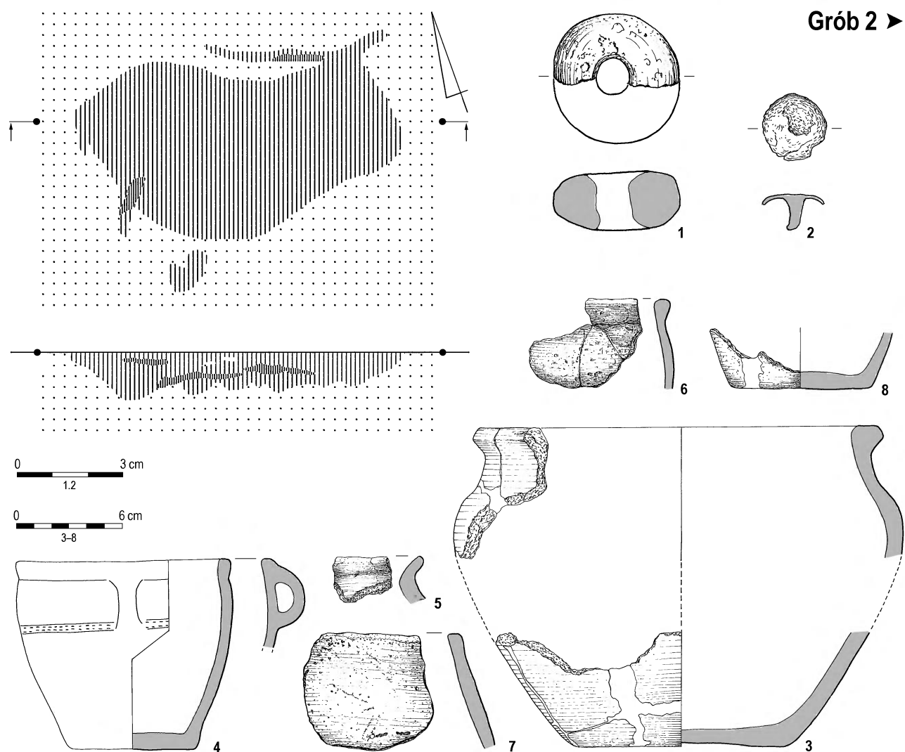
Tabl. II. Całowanie, pow. otwocki, stan. XXVI. Groby 1 i 2. 1:8-14, 2:1.3-8 – glina; 2:2 – żelazo. Rys. B. Karch Pl. II. Całowanie, distr. Otwock, site XXVI. Graves 1 and 2. 1:8-14, 2:1. 3-8 – pottery; 2:2 iron. Drawn by B. Karch
