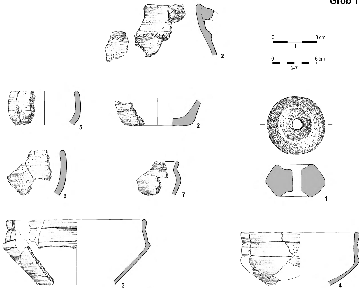
Tabl. VIII. Całowanie, pow. otwocki, stan. XXVI. Groby 10, 11 i 13. Wszystko glina. Rys. B. Karch Pl. VIII. Całowanie, distr. Otwock, site XXVI. Graves 10, 11 and 13. Pottery. Drawn by B. Karch
