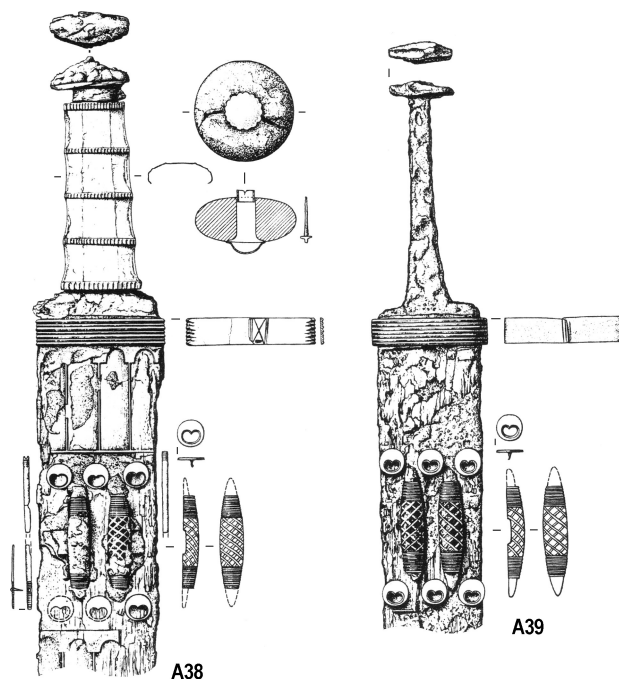
Ryc. 8. Przykłady zawieszek pochwy miecza typu Hemmingen-Pleidelsheim z Basel-Kleinhüningen, Kr. Basel.
