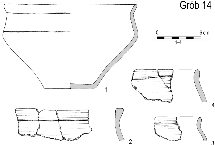
Ryc. 12. Zgliczyn Pobodzy, pow. żuromiński. Groby 13 i 14. 14/1–4 – glina. Rys.: B. Karch Fig. 12. Zgliczyn Pobodzy, Żuromin County. Graves 13 and 14. 14/1–4 – clay. Drawing: B. Karch
