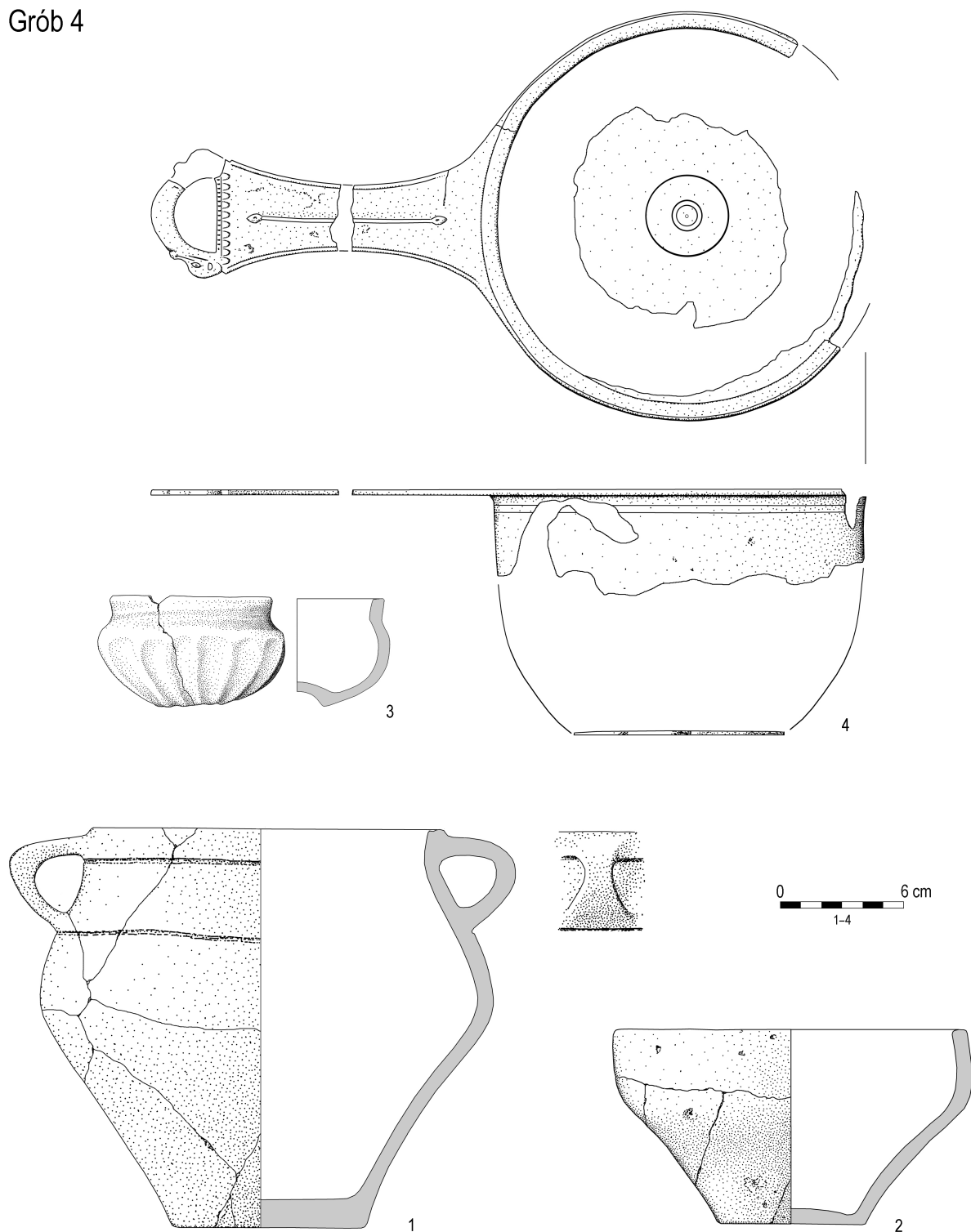
Ryc. 8. Zgliczyn Pobodzy, pow. żuromiński. Inwentarz grobu 4. 4/1-3 – glina, 4/4 – brąz. Wg: J. Schuster 2016 Fig. 8. Zgliczyn Pobodzy, Żuromin County. Equipment of grave 4. 4/1-3 – clay, 4/4 – bronze. After: J. Schuster 2016
