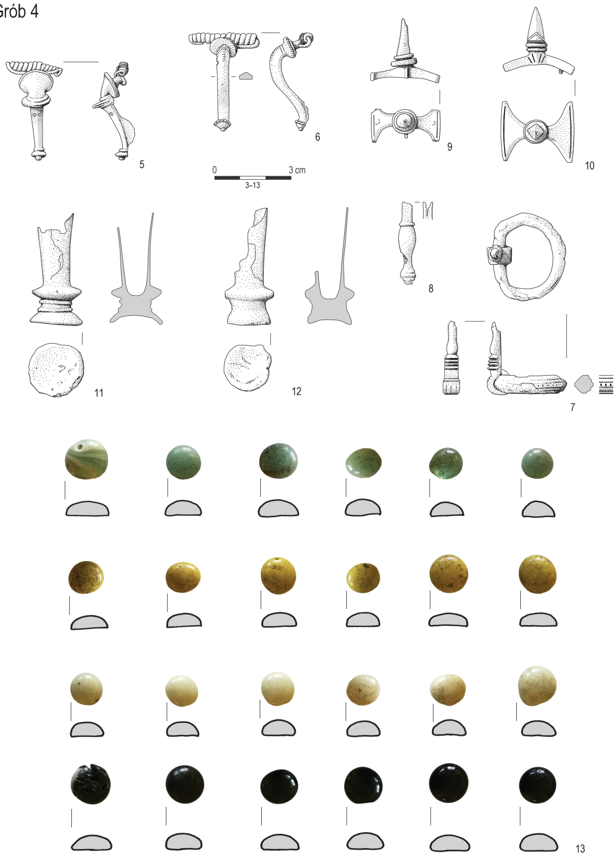
Ryc. 9. Zgliczyn Pobodzy, pow. żuromiński. Inwentarz grobu 4. 4/5.6.8-12 – brąz, 4/7 – żelazo, 4/13 – szkło.
