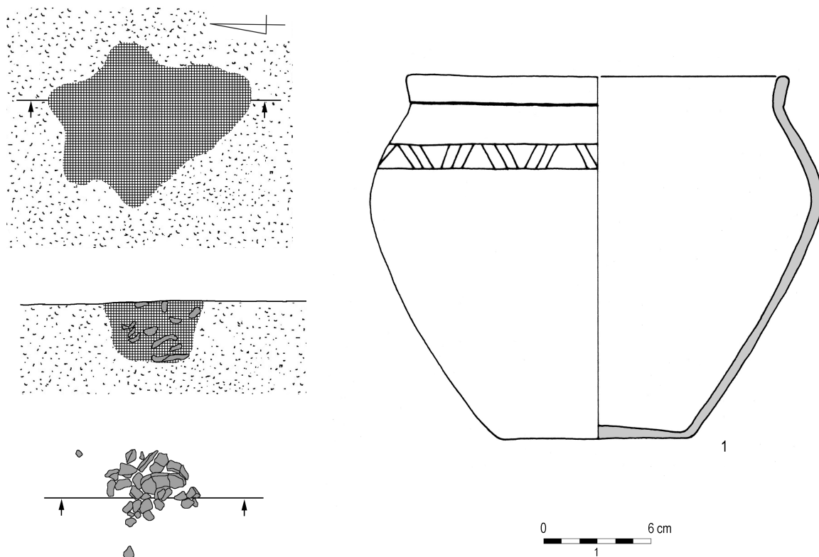
Ryc. 5. Zgliczyn Pobodzy, pow. żuromiński. Grób 3. 3/1 – glina. Rys.: B. Karch Fig. 5. Zgliczyn Pobodzy, Żuromin County. Grave 3. 3/1 – clay. Drawing: B. Karch
